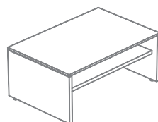
AC-MCT774D L:700 P:700 A:400 AC-MCT664D L:600 P:600 A:400 AC-MCE964D L:900 P:600 A:400 AC-MCE1064D L:1000 P:600 A:400 AC-MCE1164D L:1100 P:600 A:400 AC-MCE1264D L:1200 P:600 A:400
